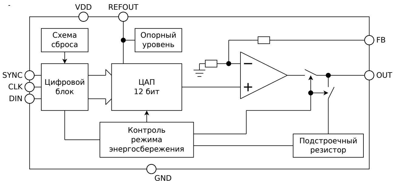
Рисунок 1. Структурная схема
