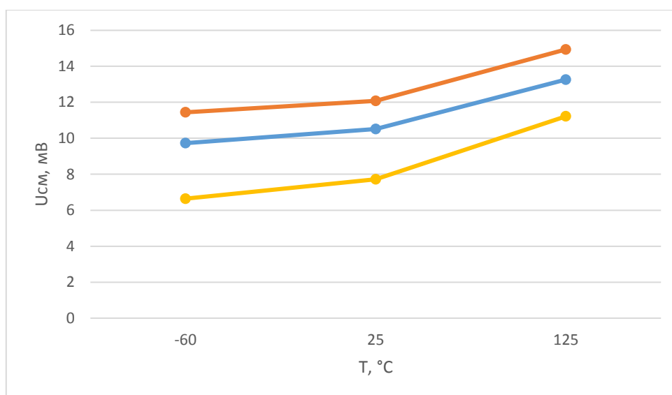
Рисунок 9. Зависимость напряжения смещения от температуры (VDDINT = 5 В)
