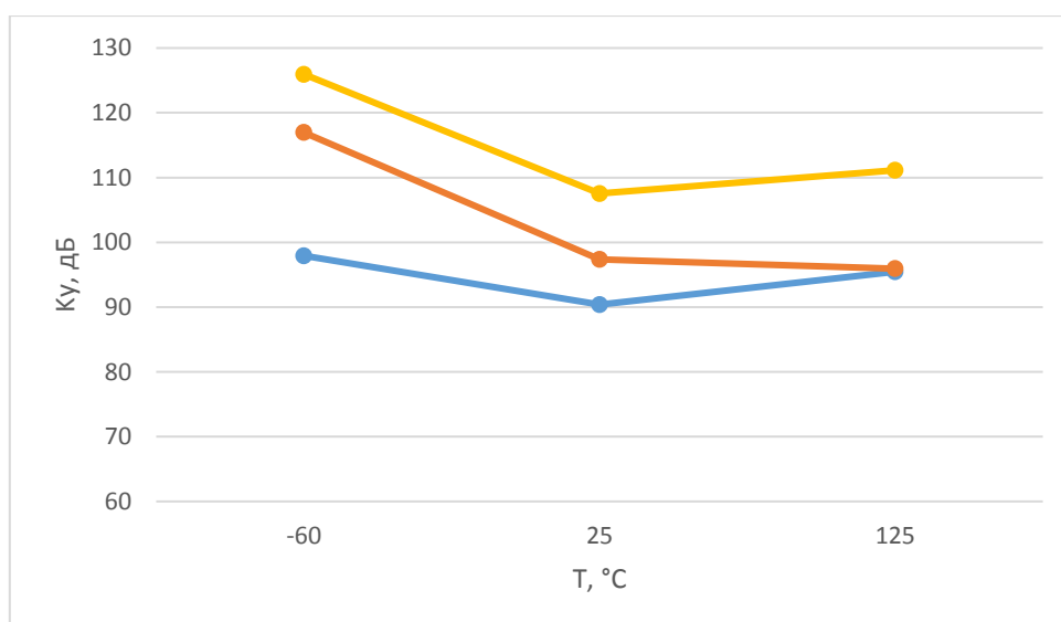
Рисунок 11. Зависимость коэффициента усиления от температуры (VDDINT = 5 В)
