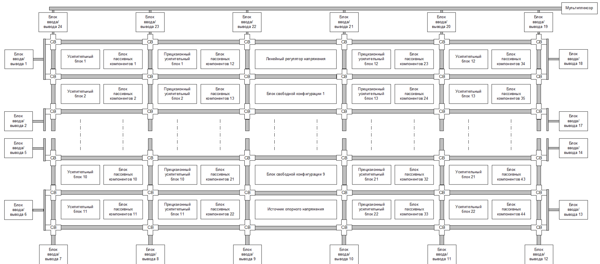
Рисунок 1. Структурная схема
